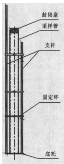
图 1 采样器结构示意图
